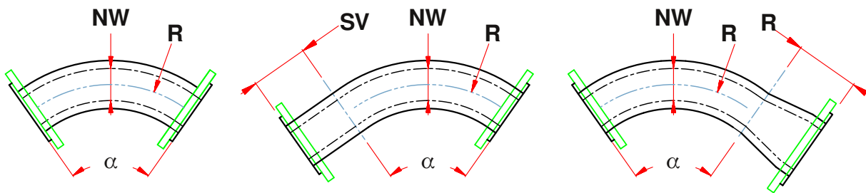
Отвод асимметричный
